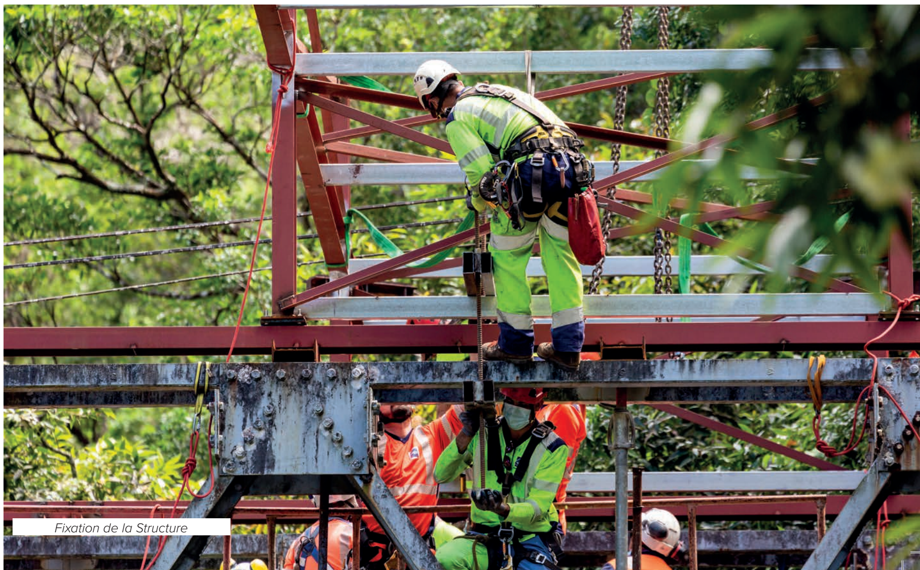
Mise en place de la Structure
